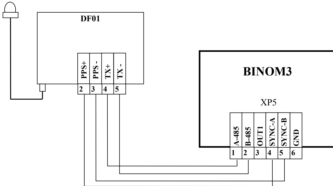
Рисунок 2.1. Стенд для определения погрешностей измерения текущего времени и приема метки синхронизации для модификаций BINOM335, BINOM336, BINOM336s, BINOM338, BINOM338s, BINOM339.
