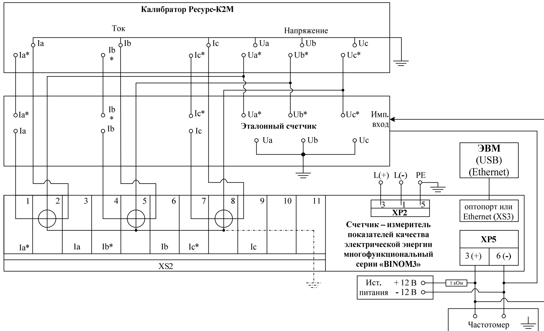
Рисунок 4 - Схема проверки счетчиков – измерителей показателей качества электрической энергии многофункциональных серии «BINOM3»
